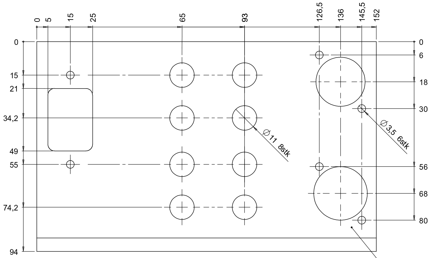
STIKPLADE. Matr.: Aluminium, eks. 3003. Blæses med Alumina til "satin" finish. Blankeloxeres. Denne forside skal fremstå ensartet, uden ridser, skygger mm.
