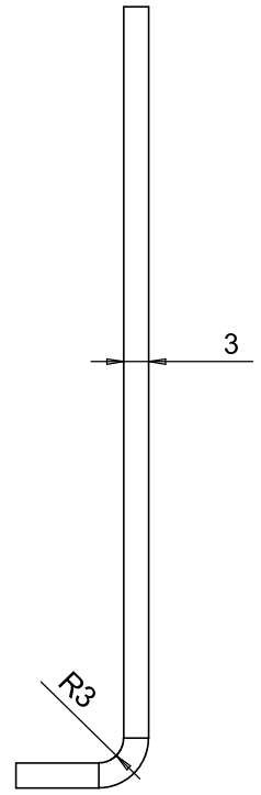
STIKPLADE. Matr.: Aluminium, eks. 3003. Blæses med Alumina til "satin" finish. Blankeloxeres. Denne forside skal fremstå ensartet, uden ridser, skygger mm.
